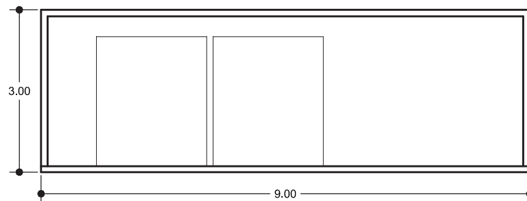
alçado principal
